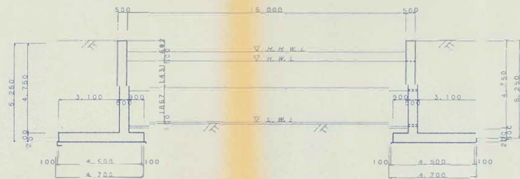
B-B 断面図 S=1:100
