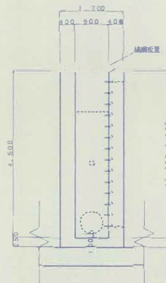
B-B 断面図 S=1:50
