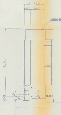
A-A 断面図 S=1:50
