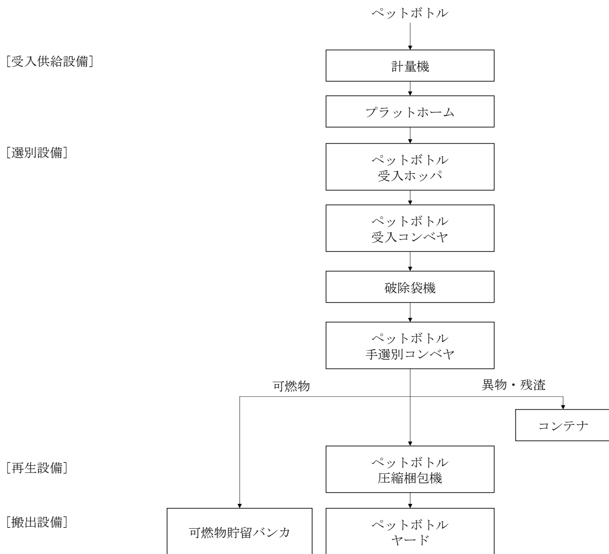
図 2.1-1③ ペットボトル処理施設の基本処理フロー（参考）
