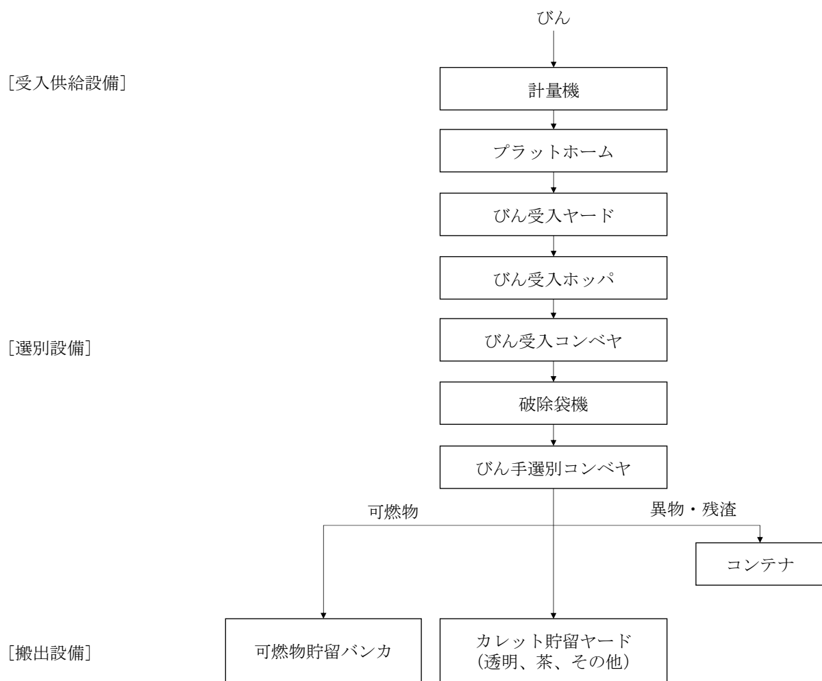
図 2.1-1④ びん処理施設の基本処理フロー (参考)
