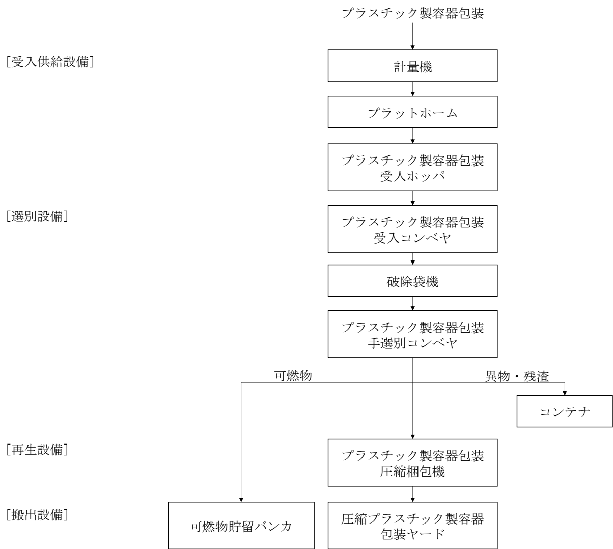
図 2.1-1② プラスチック製容器包装処理施設の基本処理フロー（参考）
