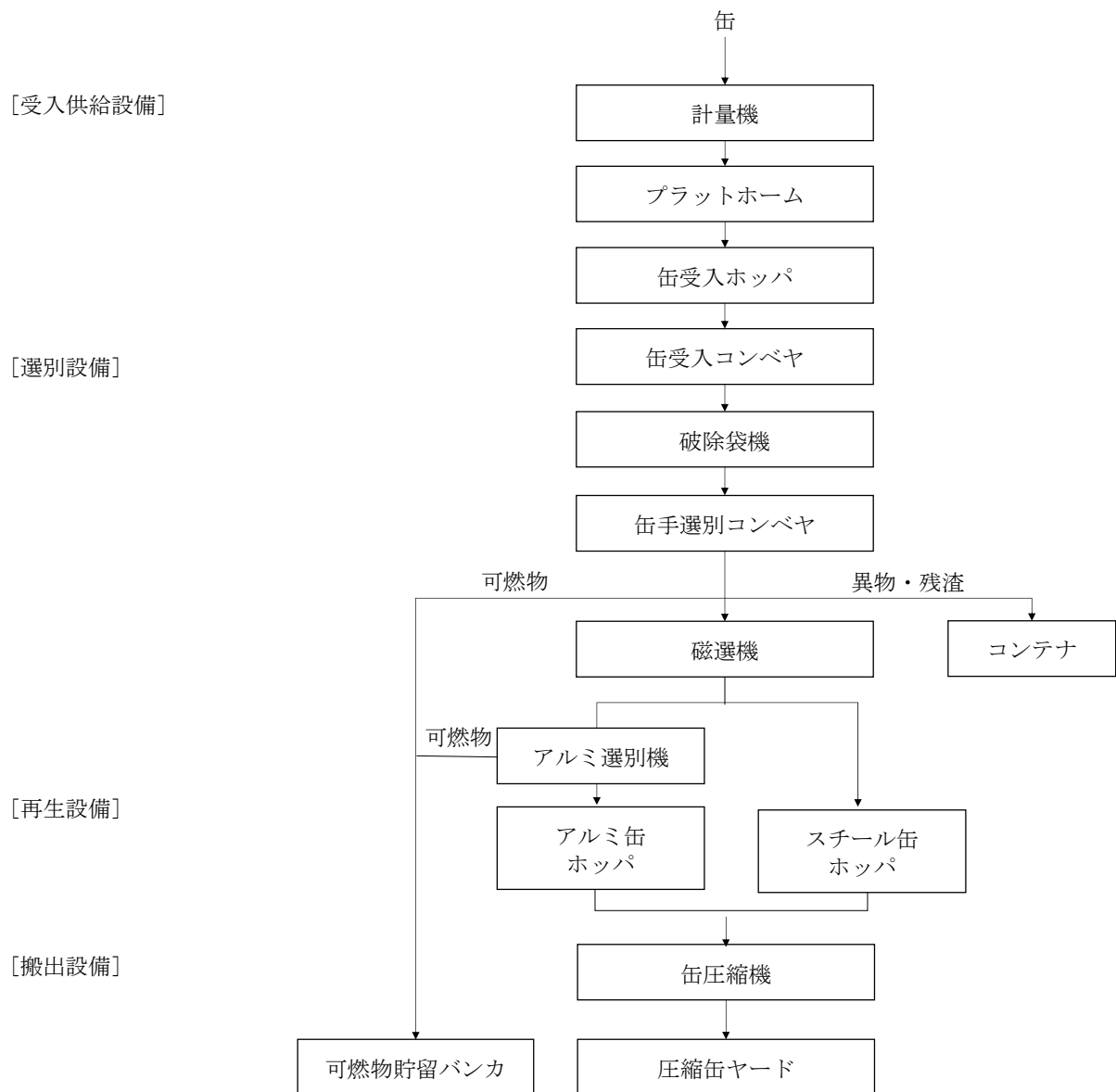
図 2.1-1⑤ 缶処理施設の基本処理フロー（参考）
