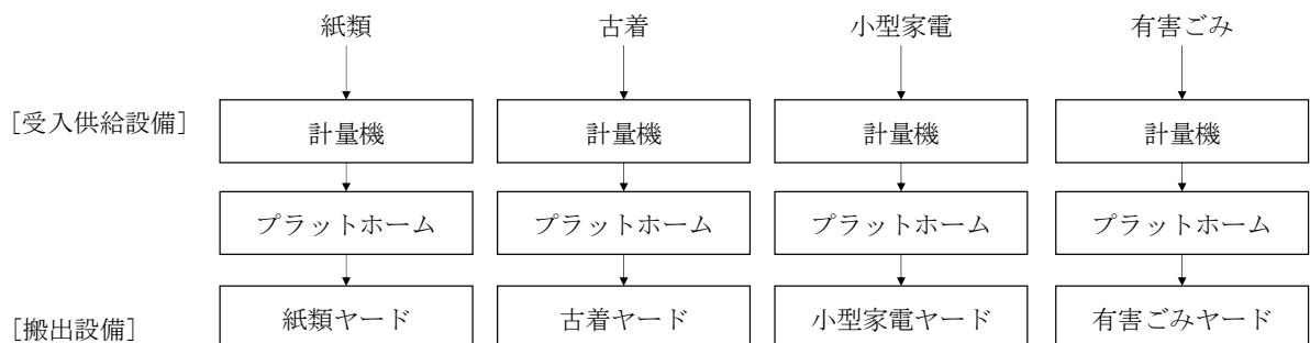
図 2.1-1⑥ その他（紙類、古着、小型家電、有害ごみ）の基本処理フロー（参考）
