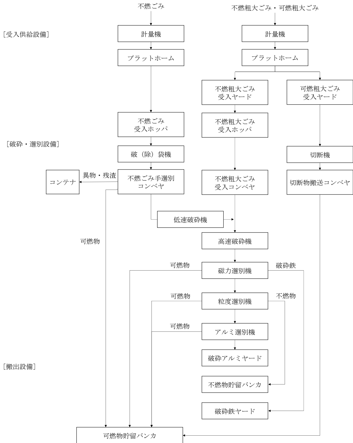
図 2. 1-1① 不燃ごみ・粗大ごみ処理施設の基本処理フロー (参考)
