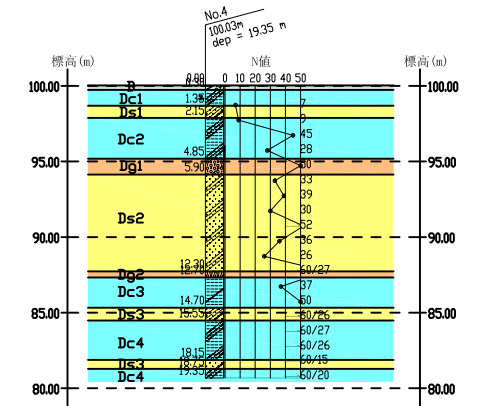
想定断面図 縮尺A3 1:500
