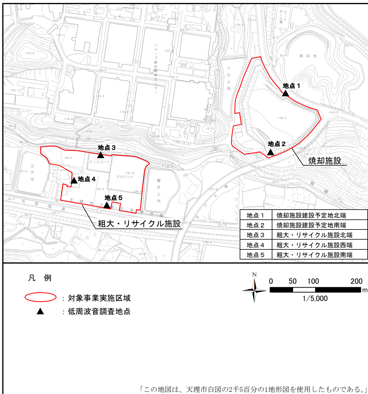
図 7.2-7 低周波音の調査地点
