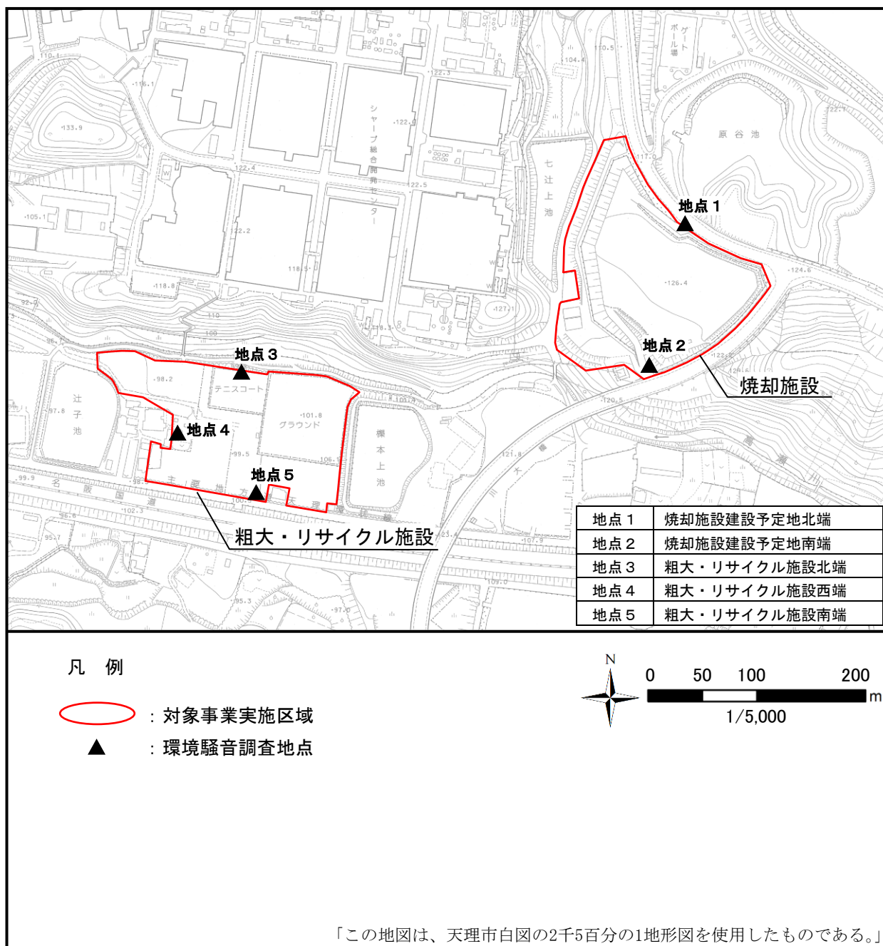
図 7.2-3 環境騒音の調査地点
