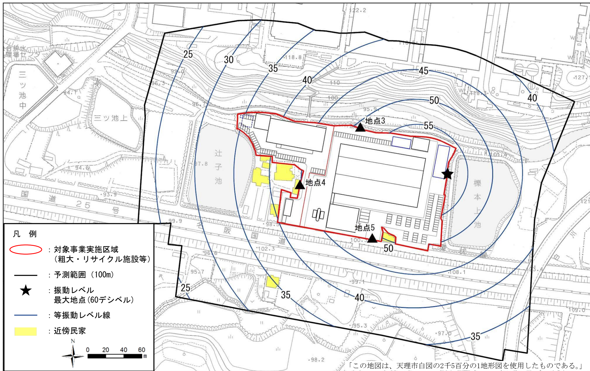
図 7.3-12 施設の稼働に伴う振動の予測結果 (粗大・リサイクル施設等)
